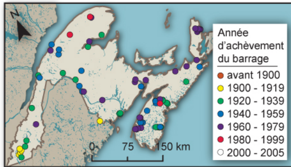
Figure 17. Répartition spatiale des barrages de plus de 10 m de haut dans l'écozone + maritime de l'Atlantique, groupés par année d'achèvement entre 1830 et 2005.
