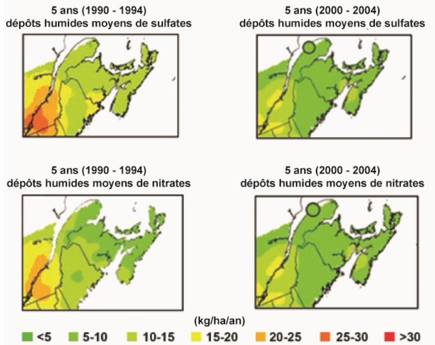
Figure 35. Tendence des dépôts humides de sulfates et de nitrates dans l'écozone + maritime de l'Atlantique durant les périodes 1990-1994 et 2000-2004.
